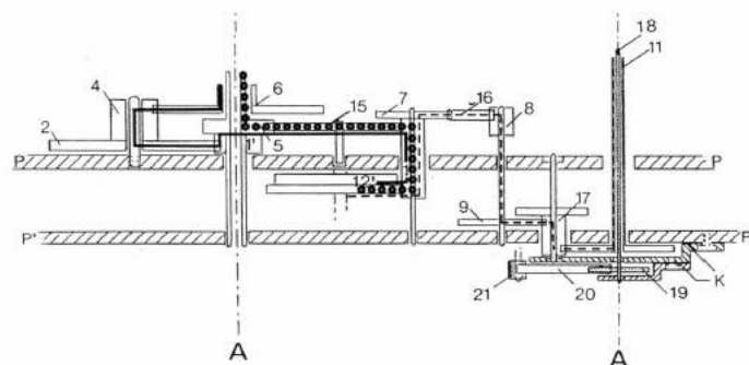
13f Schnitt-Skizze durch das Zeigerwerk der 95656. Die Kraftflußwege zu den Zeigern sind markiert: durchgehende Linie → 1. Gradzeiger, groß-gepunktete Linie → 2. Gradzeiger, gestrichelte Linie → 1. Bogenminutenzeiger, klein-gepunktete Linie → 2. Bogenminutenzeiger (Schleppzeiger)
