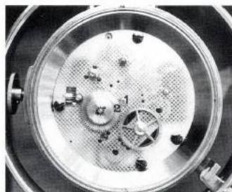
8d Weitere Abnahme des 2. Gradzeigerrades [5] und 1. Bogenminutenrades [10] mit Kloben [K]. Gut sichtbar der Eingriff vom Minutentrieb [1] in das untere Wechselrad [2]
