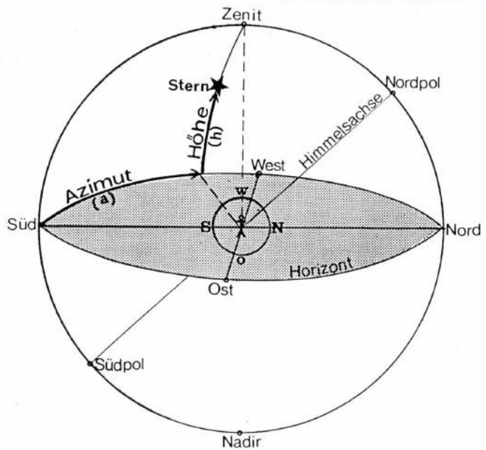
2 Himmels-Horizontalkoordinatensystem mit Azimet ( a ) = Länge am Horizont vom Südpunkt bis zum Vertikal des Gestirns und Höhe ( h ) = Breite vom Horizont auf dem Vertikal bis zum Gestirn in Richtung Zenit
