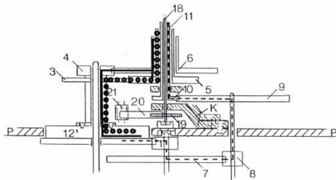
13f Schnitt-Skizze durch das Zeigerwerk der 95656. Die Kraftflußwege zu den Zeigern sind markiert: durchgehende Linie → 1. Gradzeiger, groß-gepunktete Linie → 2. Gradzeiger, gestrichelte Linie → 1. Bogenminutenzeiger, klein-gepunktete Linie → 2. Bogenminutenzeiger (Schleppzeiger)
