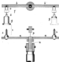
Abb. 1. Die „Glockenhemmung“ vermeidet die Fadenaufhängung der Gewichte
